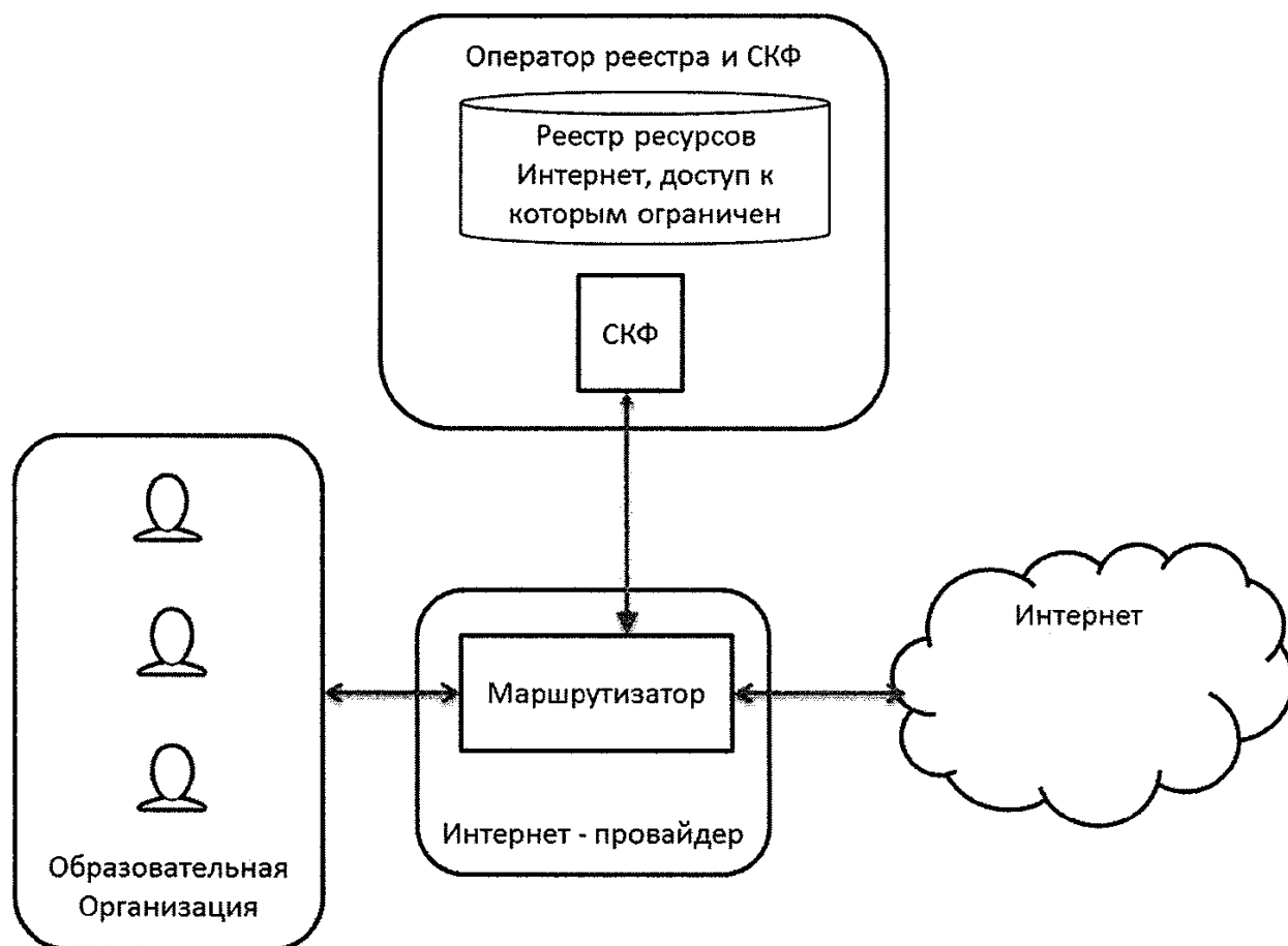
Рисунок 5. Схема работы контент-фильтрации при едином решении
